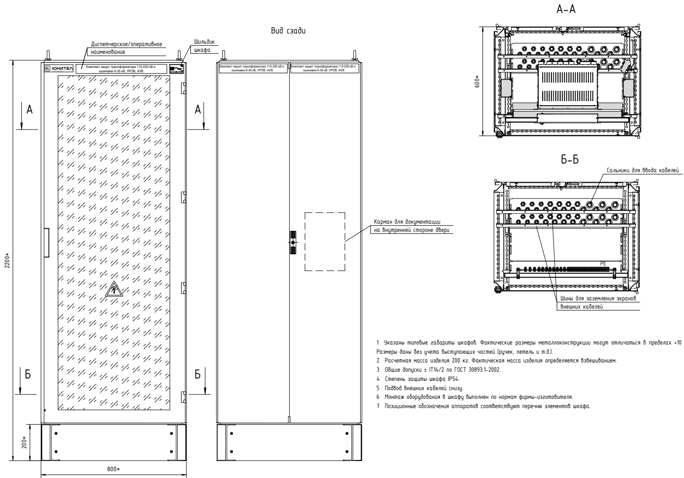
Рисунок Б.1 – Чертеж общего вида (часть 1)
